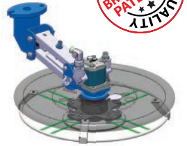
Sistema BREVETTATO di fissaggio del filo Wire fixing PATENTED system PATENTIERTES System zur Drahtbefestigung Sistema PATENTADO de fijación de hilo Système BREVETÉ de fixation du fil
